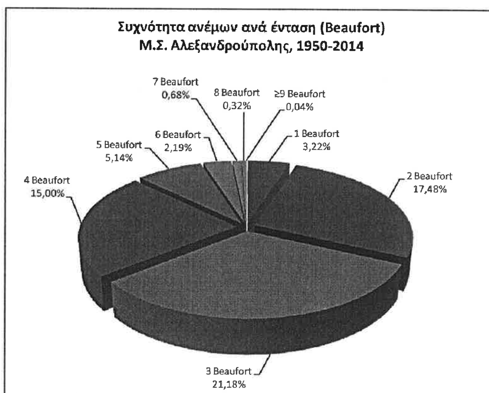
Εικόνα 5. Κατανομή ανέμων (%) ανά κλίμακα έντασης (Beaufort) Μ.Σ. Αλεξανδρούπολης (περίοδος 1950-2014)
