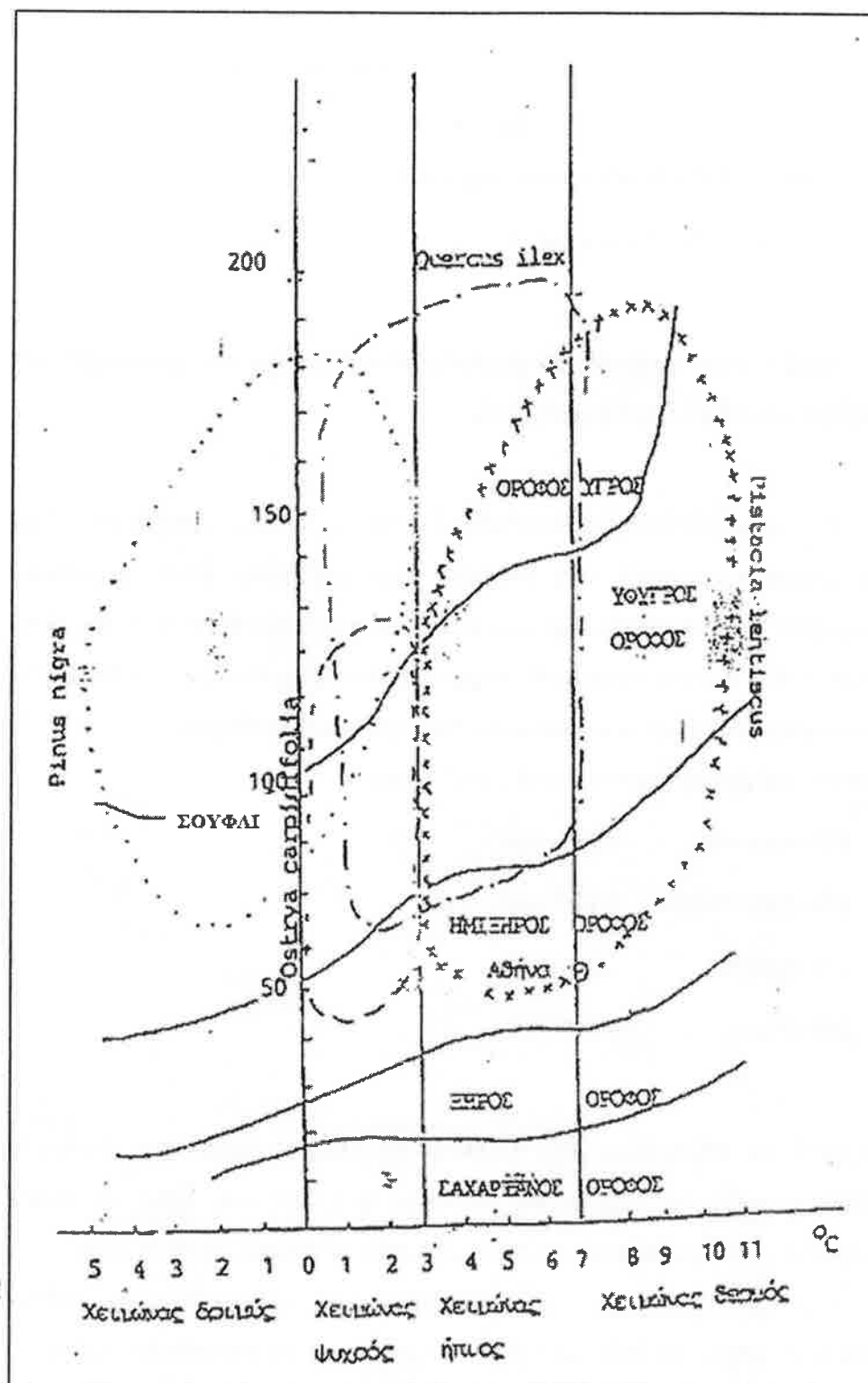
Εικόνα 6. Κλιματικό διάγραμμα Emberger για την περιοχή του Μ. Σ. Σουφλίου
