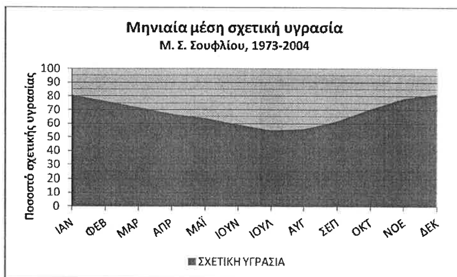
Εικόνα 3. Μηνιαία μέση σχετική υγρασία Μ.Σ. Σουφλίου (περίοδος 1973-2004)
