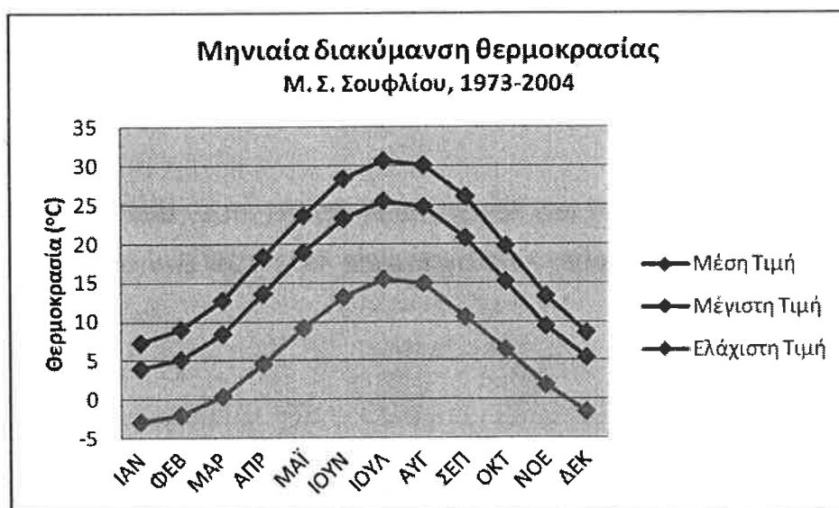
Εικόνα 1. Μηνιαία διακύμανση θερμοκρασίας Μ.Σ. Σουφλίου (περίοδος 1973-2004)
