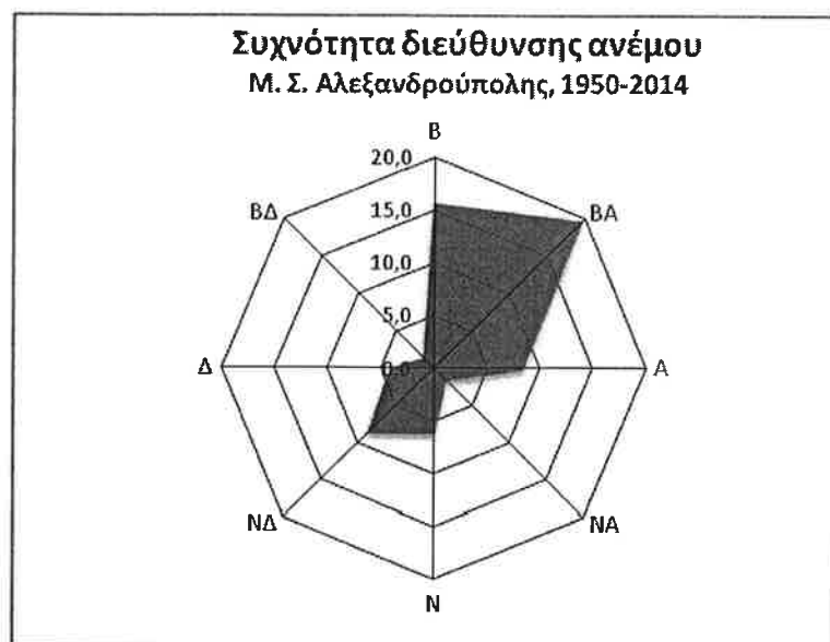
Εικόνα 4. Ανεμολογικό διάγραμμα Μ.Σ. Αλεξανδρούπολης (περίοδος 1950-2014)
