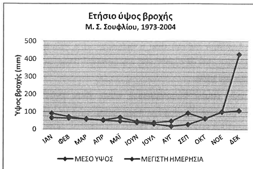
Εικόνα 2. Ετήσιο ύψος βροχής Μ.Σ. Σουφλίου (περίοδος 1973-2004)
